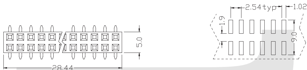
P.C.B Layout
