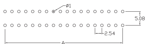
P.C.B Layout
