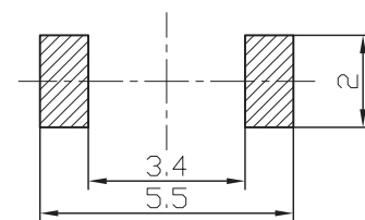
安装参考尺寸 P.C.B layout
