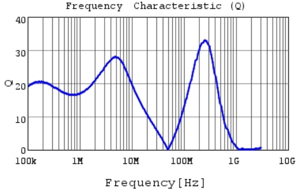
LQH5BPN4R7NT0 Q
