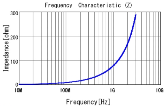
■ LQW15AN12NG00 |Z|
