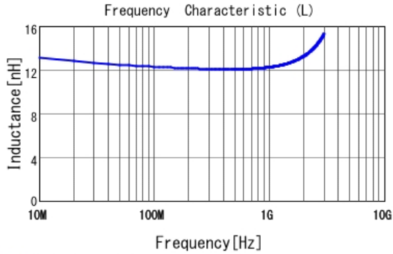
■ LQW15AN12NG00 L
