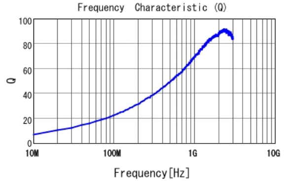
■ LQW15AN12NG00 Q
