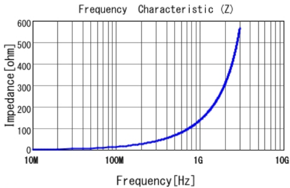
■ LQW15AN22NG00 |Z|
