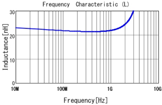
■ LQW15AN22NG00 L
