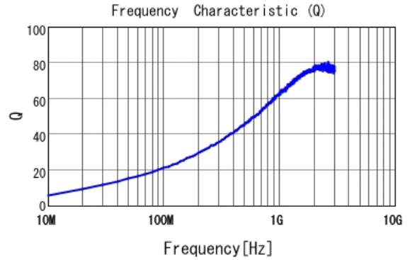
■ LQW15AN22NG00 Q
