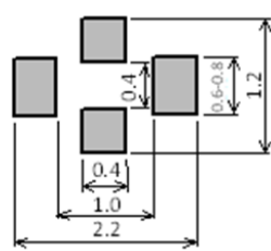
NFM18HC105
