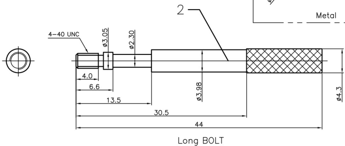
Long BOLT
